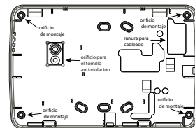
Figura 2 – Montaje de la placa de apoyo
