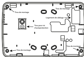
Figure 2 : Montage de la plaque arrière
