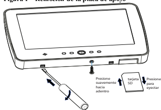
Figura 1 – Remoción de la placa de apoyo
