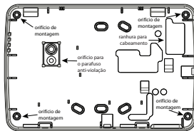
Imagem 2 – Montagem da Tampa traseira
